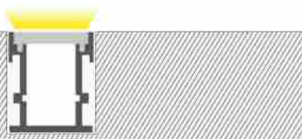
地面嵌入式安装 embedded installation
