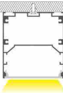
吸顶式安装 Ceiling mount
